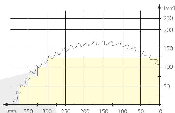
Řezný diagram pro Crossline 500
