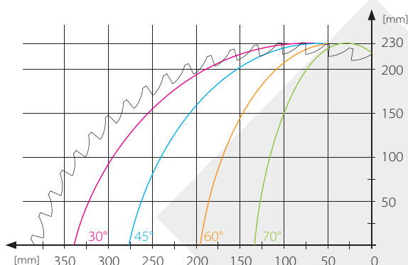
Řezný diagram pro Crossline 650
